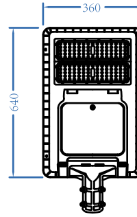
AN-ISSL-C-60W
