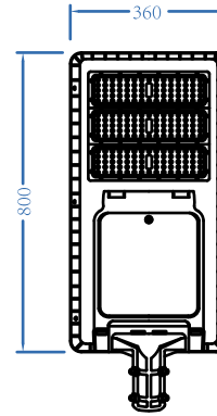
AN-ISSL-C-80W
